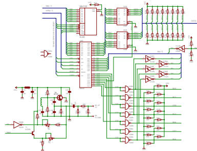
UF MODULATOR, NASOBICKA, PARALELNI MEZISTYKY
